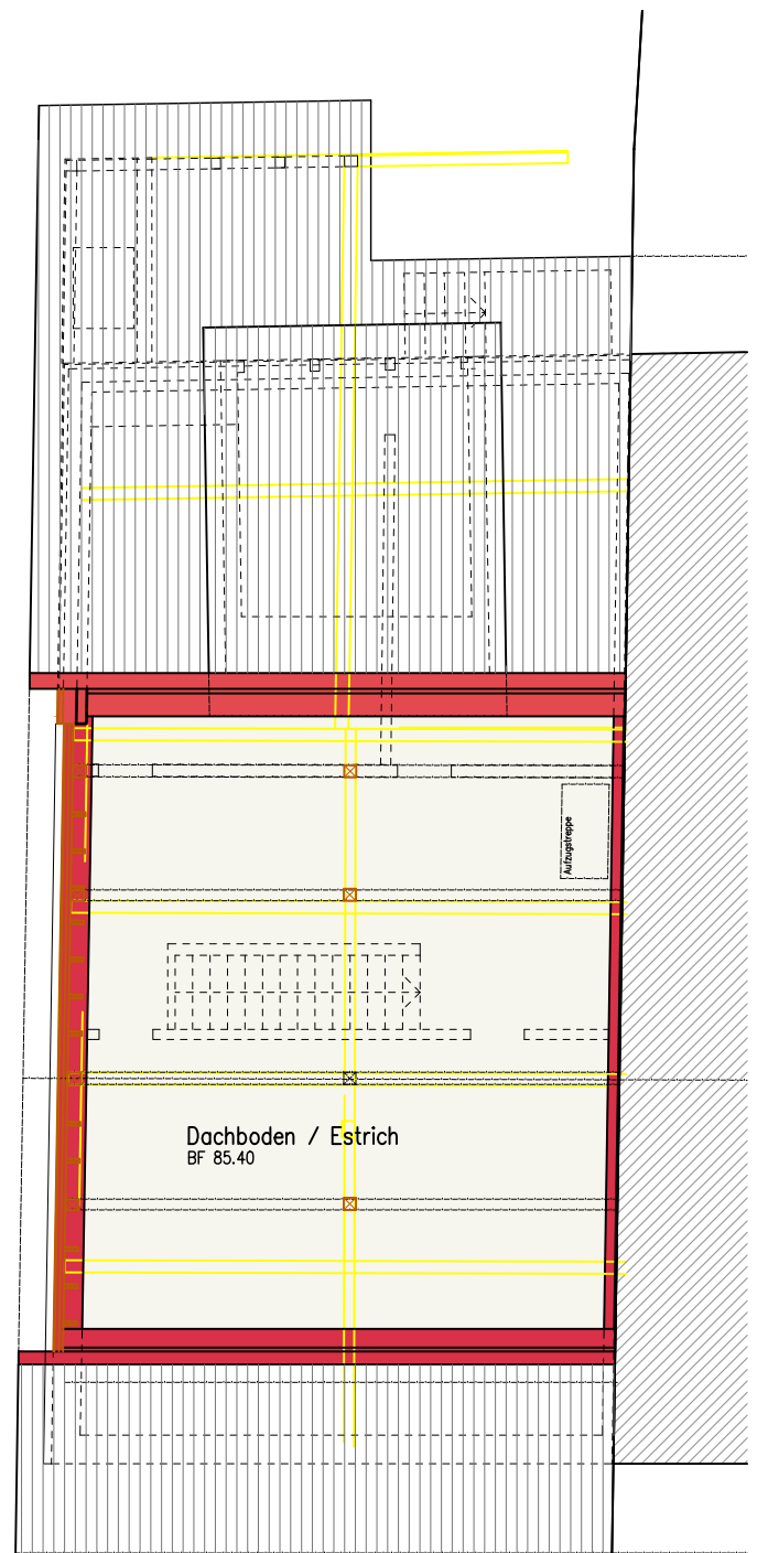
Dachgeschoss
