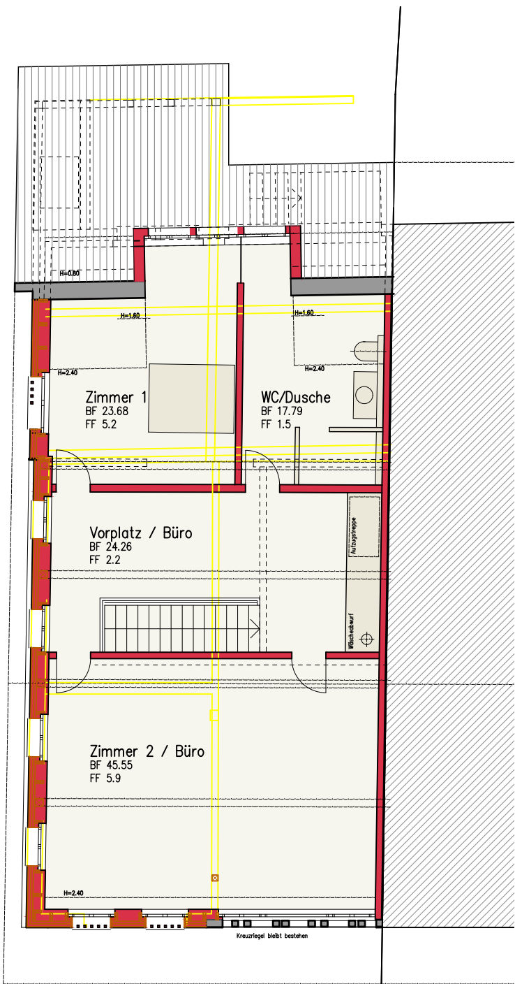
Obergeschoss
