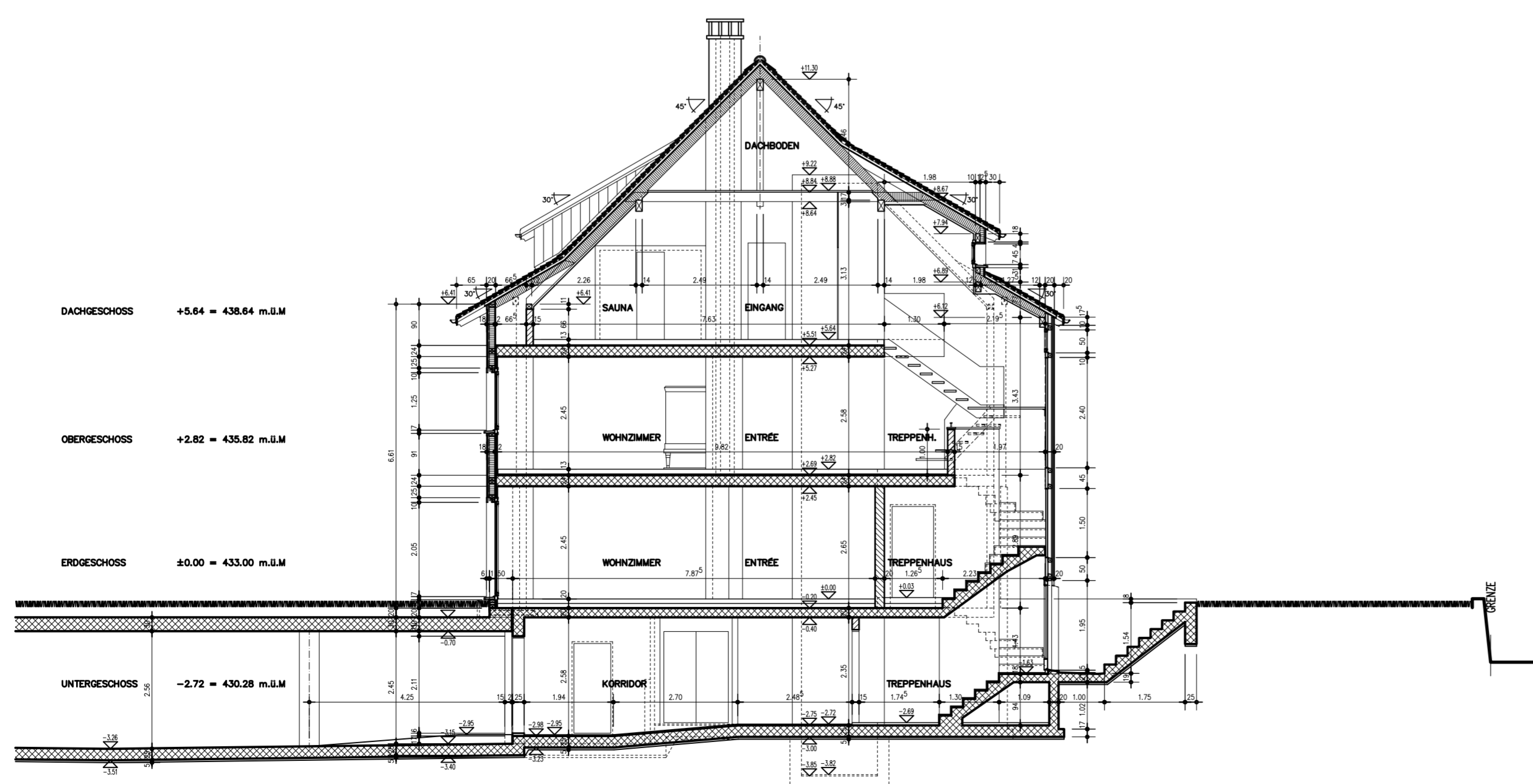
QUERSCHNITT A-A
