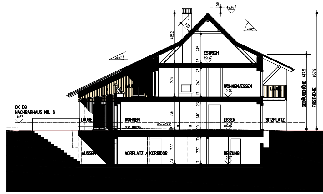
SCHNITT A-A
